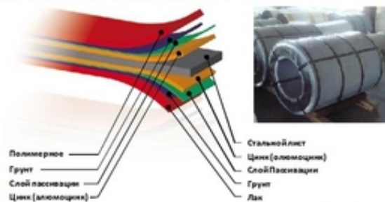
Структура листовой стали с полимерным покрытием
