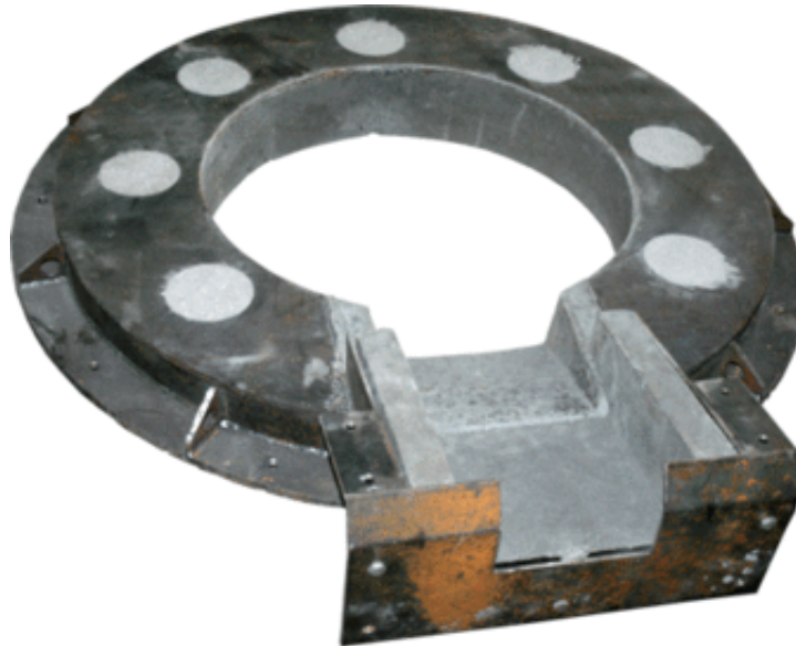
Верхняя плита в сборе ИТПЭ 1.0
